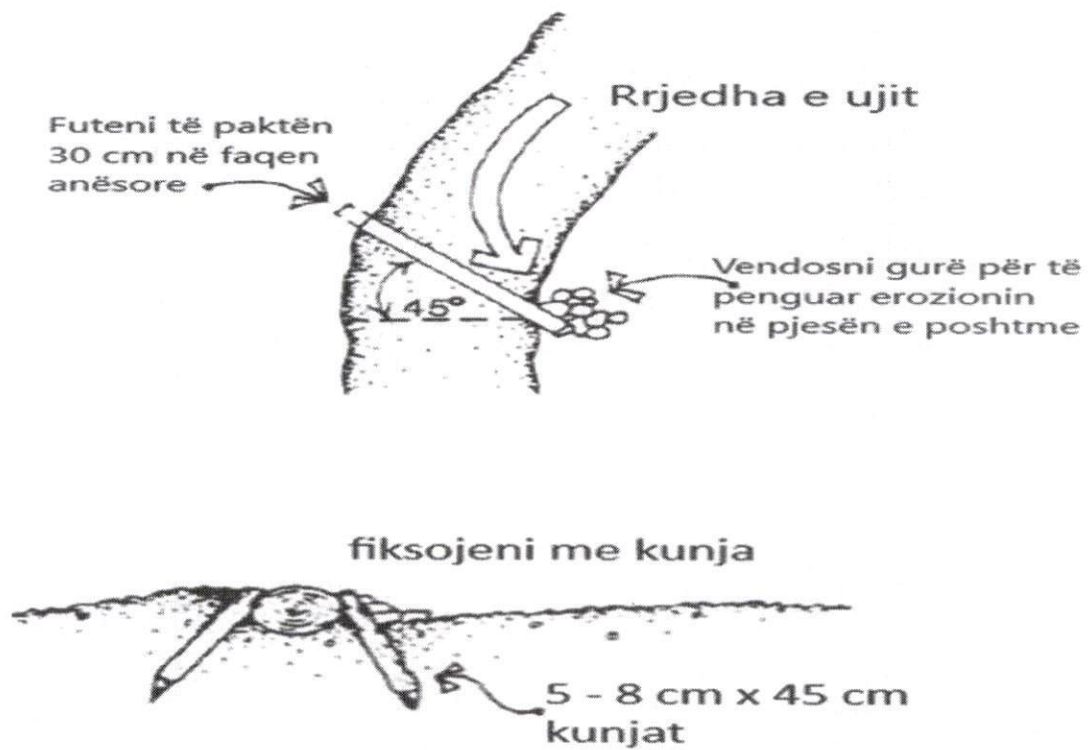
Figura 0.6 - Ujë kulluese
